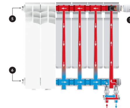
Патентован прав спирателен вентил за с-ма с „Долно присъединяване“
