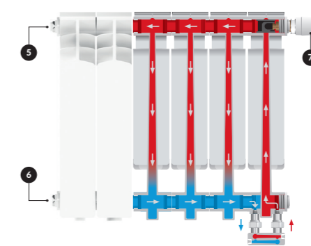
Патентован ъглов спирателен вентил за с-ма с „Долно присъединяване“
