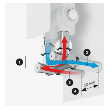
Патентован ъглов спирателен вентил за с-ма с „Долно присъединяване“
