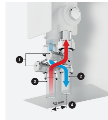
Патентован прав спирателен вентил за с-ма с „Долно присъединяване“
